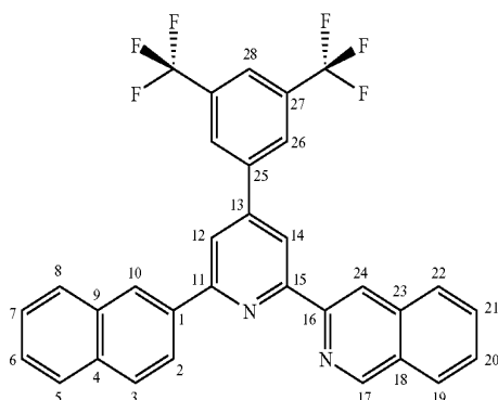
Ligand 6
