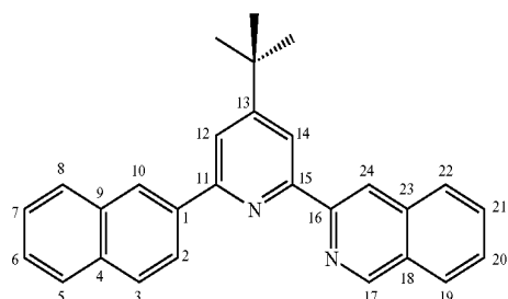
Ligand 2
