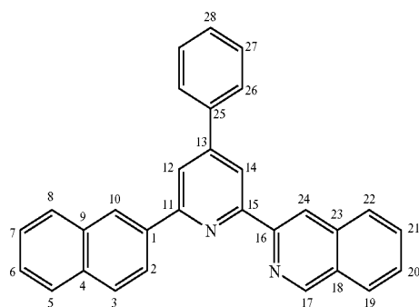
Ligand 3
