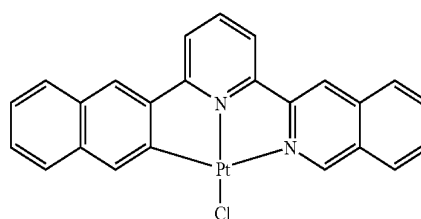
Ligand 6
