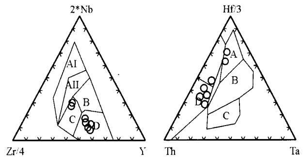
图9 塔尔浪辉长岩 Zr-Nb-Y 判别图(Meschede, 1986)和 Hf-Th-Ta 判别图(Wood, 1980)(其中 Zr-Nb-Y 判别图中: A I 区为板内碱性玄武岩, A II 区为板内碱性玄武岩和板内拉斑玄武岩, B 区为 E 型 MORB, C 区为板内拉斑玄武岩和火山弧玄武岩, D 区为 N 型 MORB 玄武岩和火山弧玄武岩。其中 Hf-Th-Ta 判别图中, A 区为 N 型 MORB, B 区为火山弧玄武岩, C 区为板内碱性玄武岩, D 区为岛弧拉斑玄武岩( Hf/Th > 3.0 )和钙碱性玄武岩( Hf/Th < 3.0 ))
