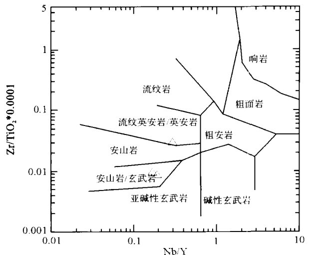
图 5 塔尔浪斜长角闪岩 Zr/TiO 2 -Nb/Y 图解 (Winchester and Floyd, 1976)
