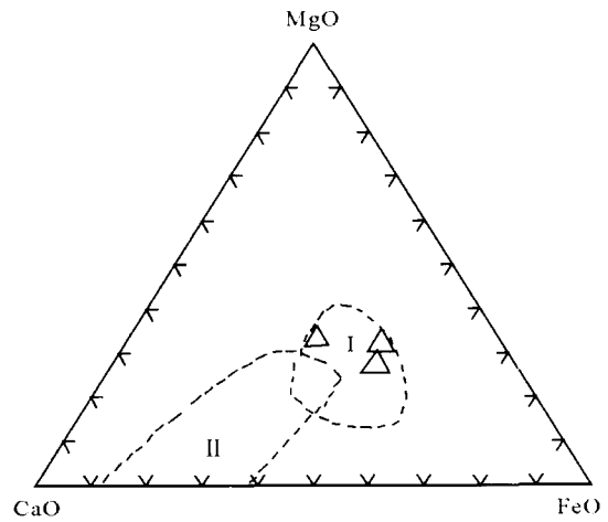
图 4 塔尔浪斜长角闪岩 MgO-CaO-FeO (Walker et al. , 1960) (其中, I 为正斜长角闪岩; II 为负斜长角闪岩)
