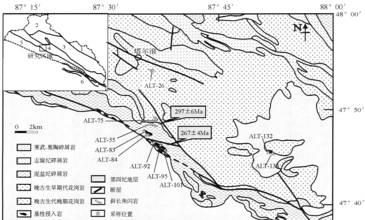
图 1 塔尔浪地区地质图
