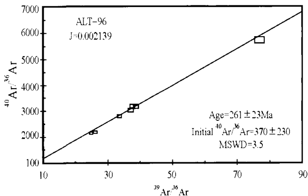
图 3 辉长岩 40 Ar- 39 Ar 等时线年龄
