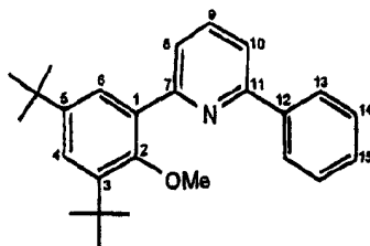
中间体 1
