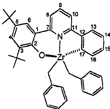
催化剂 1
