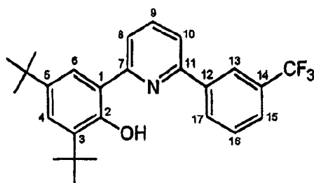
中间体 4
