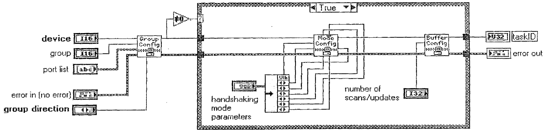
Fig. 14A : VI diagram of DIO CONFIG.vi
