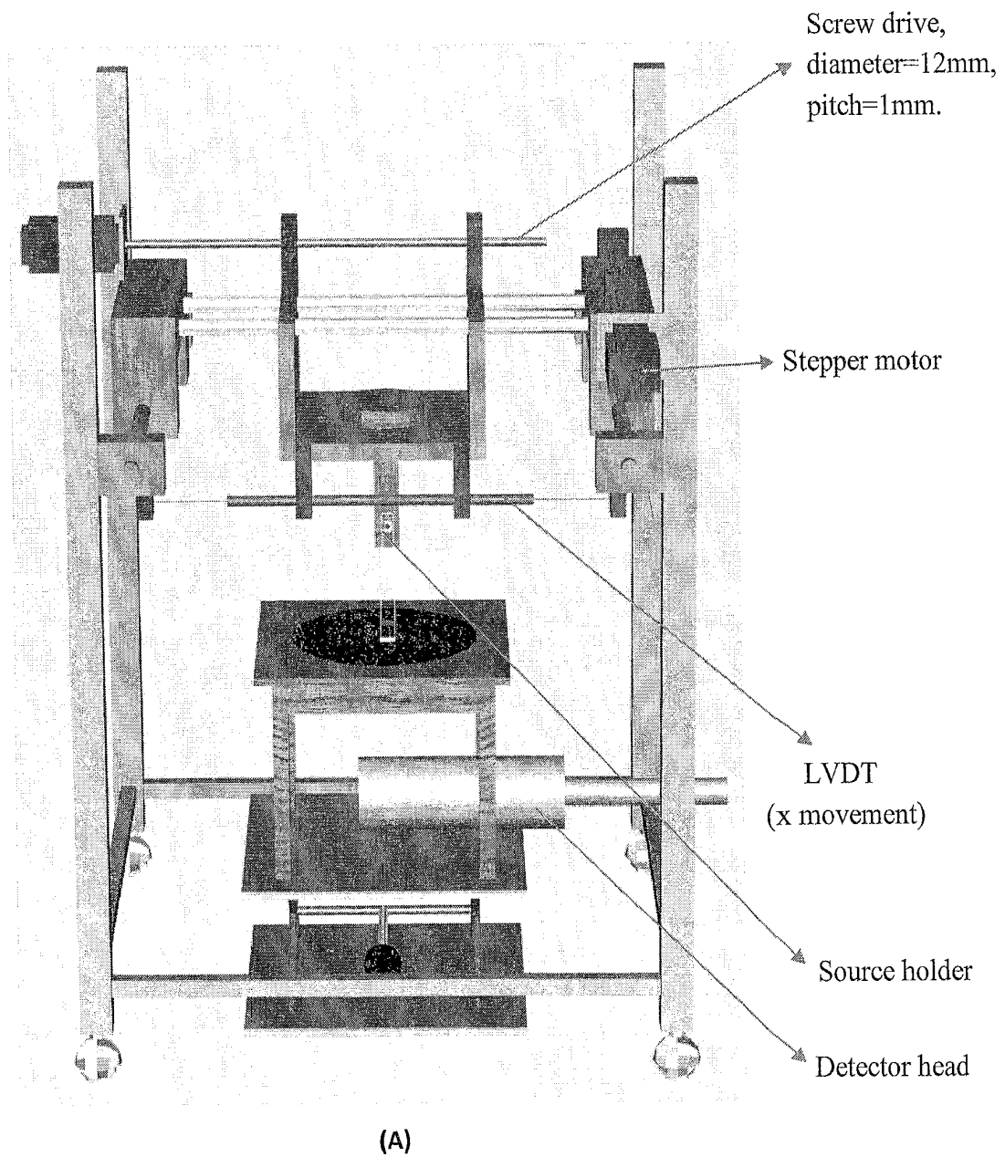
Fig-13 : Scanning apparatus : Side view.
