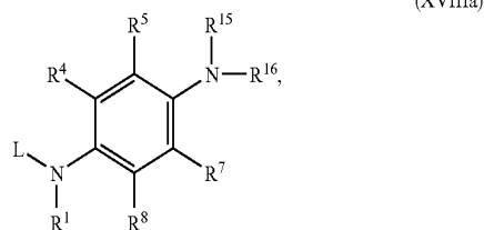
(XVIIIb)
