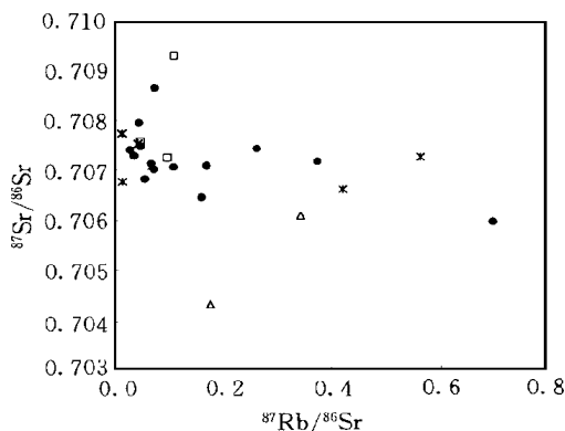
图 1 ^{87}\text{Rb}/^{86}\text{Sr} 与 ^{87}\text{Sr}/^{86}\text{Sr} 的关系
