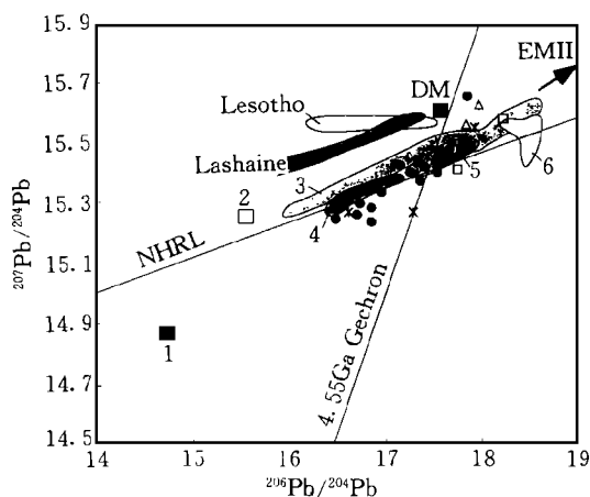
图 2 Pb 同位素组成
