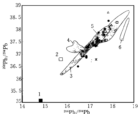
图 2 Pb 同位素组成
